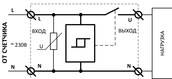
Схема подключения
